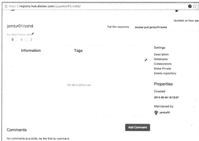
图 4-11 删除仓库
