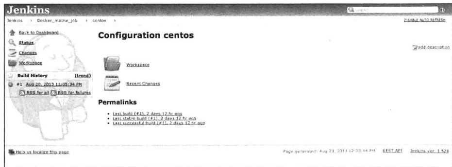
图 5-14 centos 子作业
