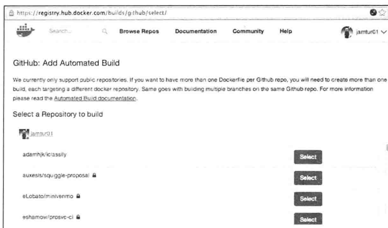
图 4-8 选择仓库
