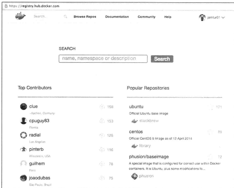
图 4-2 Docker Hub
