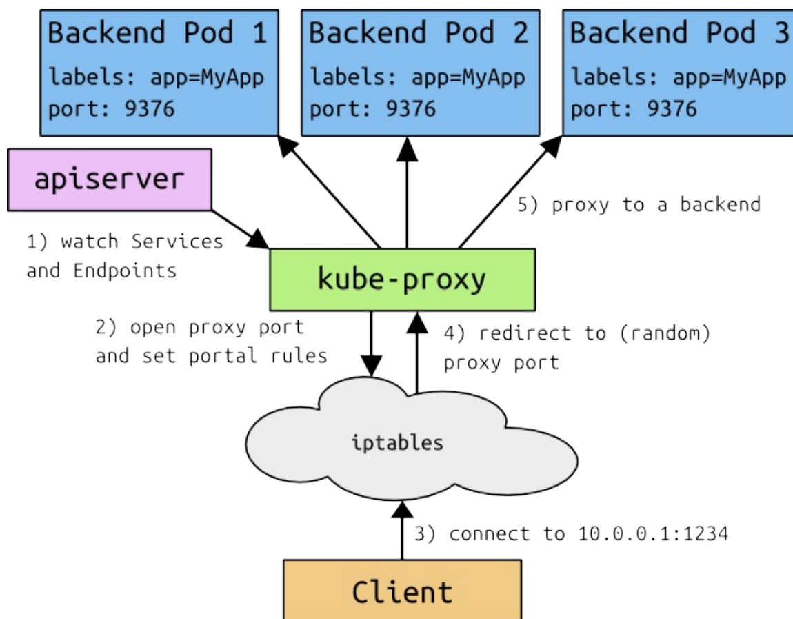
图 1.20.5.2 - Proxy 代理对服务的请求
