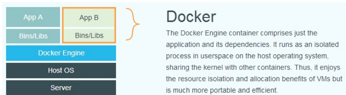
图 1.4.1.2 - Docker
