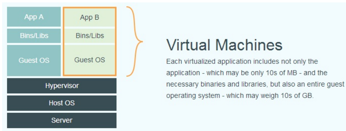
图 1.4.1.1 - 传统虚拟化
