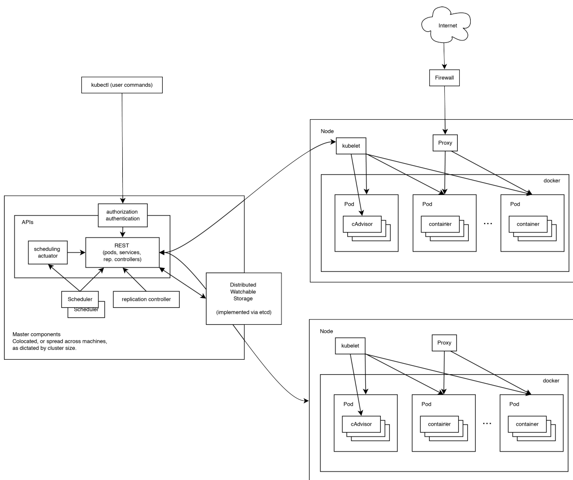
图 1.20.5.1 - Kubernetes 架构
