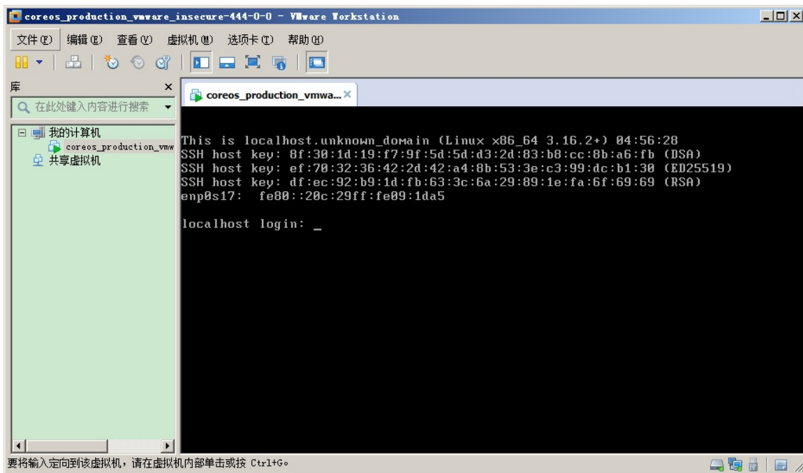
图 1.23.5.3 - 登录 CoreOS
