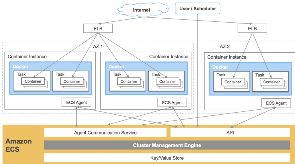
图 1.22.2.2 - AWS 容器服务
