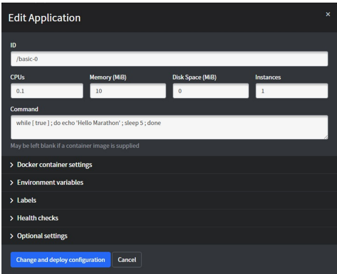
图 1.21.2.3 - marathon 查看任务支持的参数
