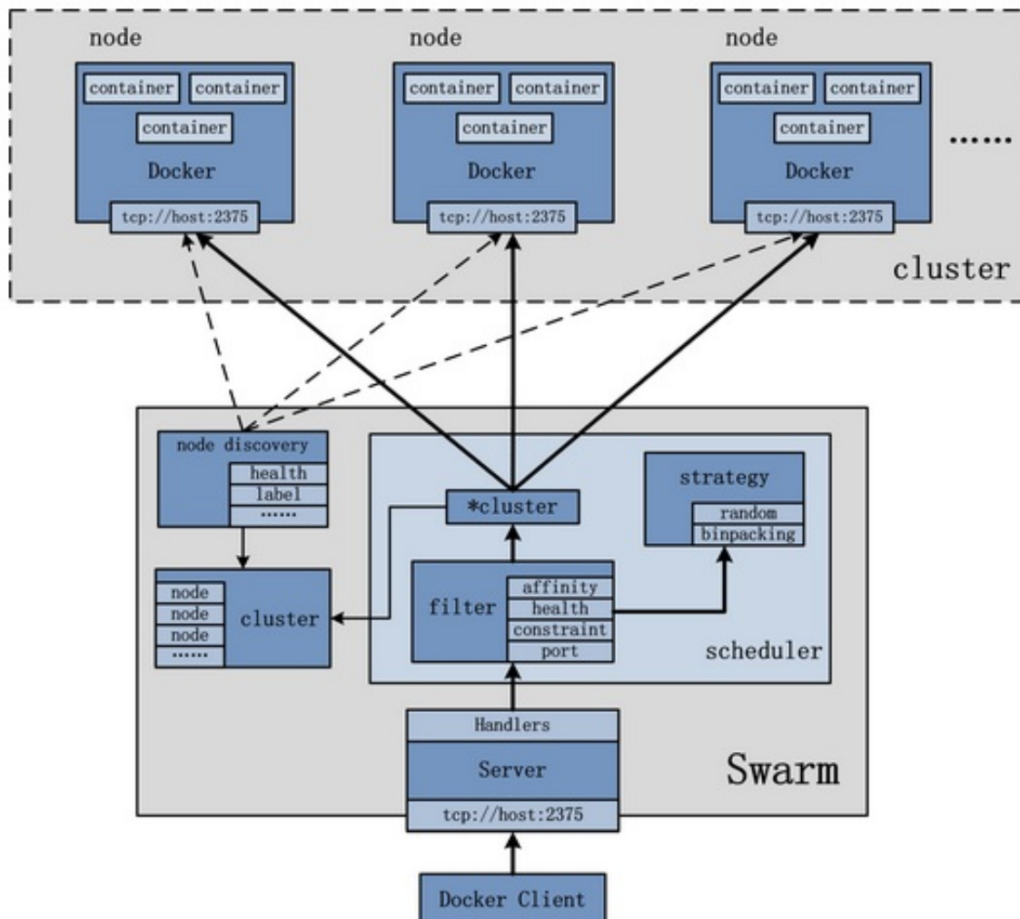
图 1.17.1.2 - Swarm 基本结构图
