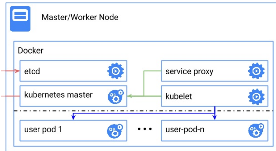
图 1.20.2.1 - 在 Docker 中启动 Kubernetes
