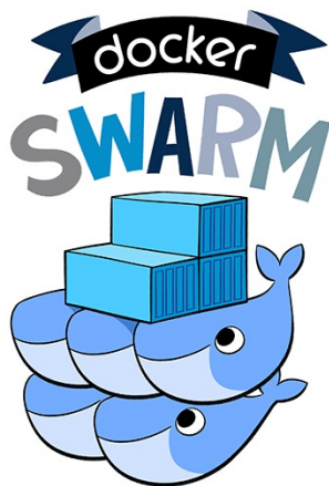
图 1.17.1.1 - Docker Swarm
